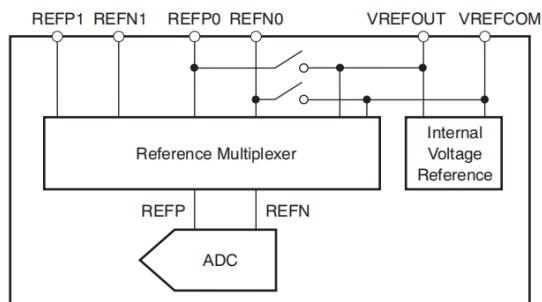
图12.参考输入复用器
