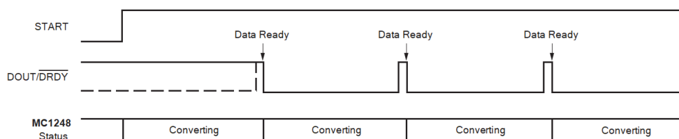
图 15. Start 引脚为高电平时的转换时序
