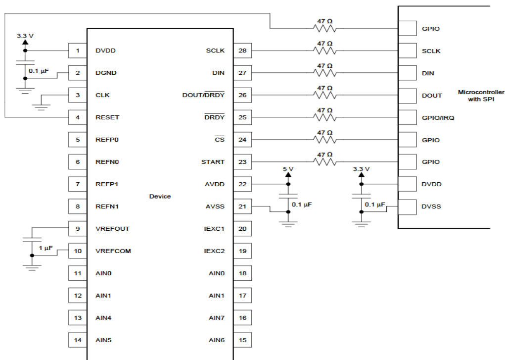
图44. 串行接口连接
