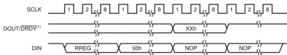
图22.读取寄存器数据后，DOUT/DRDY被强制拉高
