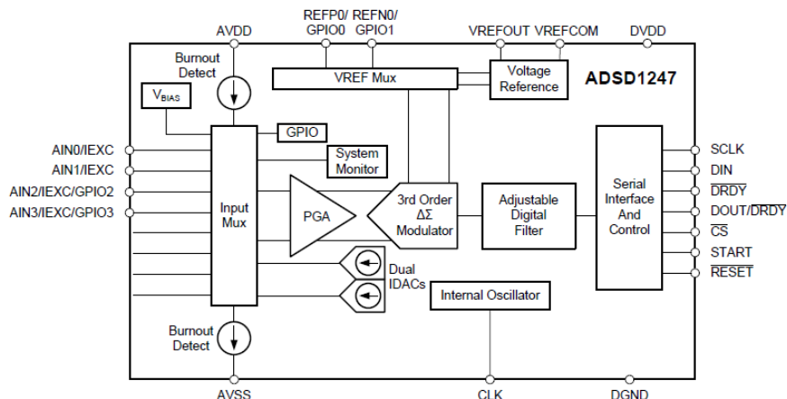
图10: 功能框图
