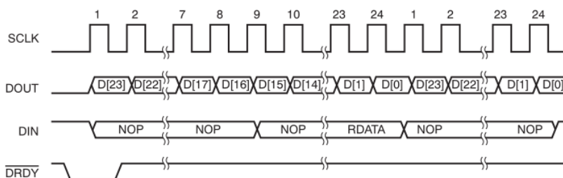
图 28.在全双工模式下使用RDATA
