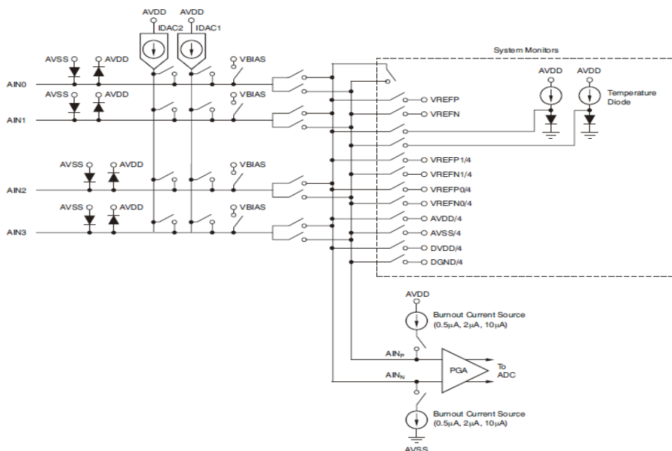
图 11.输入多路复用器简图
