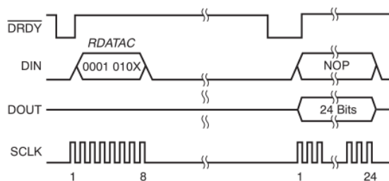
图29.连续读取数据
