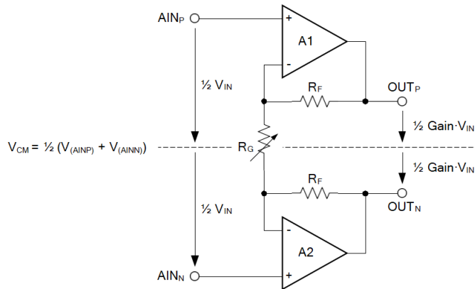
图8 .PGA 共模电压
