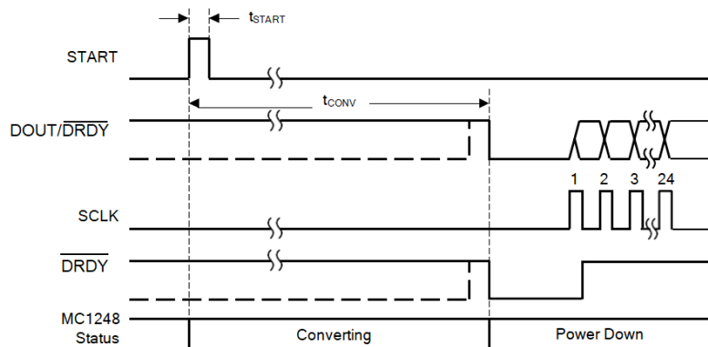
图 14. 使用 Start 引脚的单次转换时序
