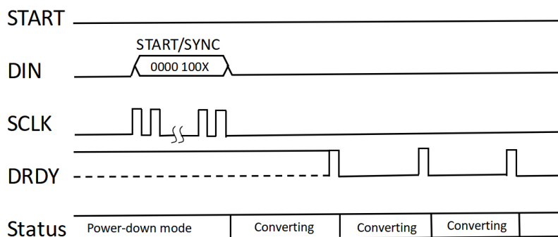
图 17.使用 START/SYNC 命令进行连续转换的时序
