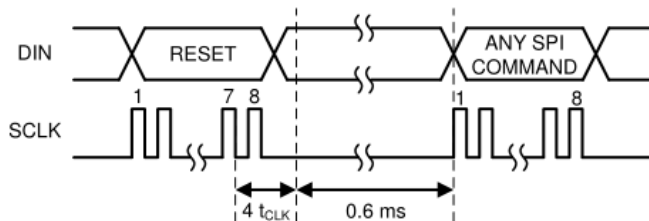
图26.SPI 复位后的SPI 通信
