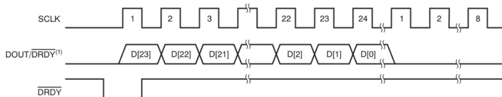
图20.DRDY模式位=0时的数据检索(禁用)
