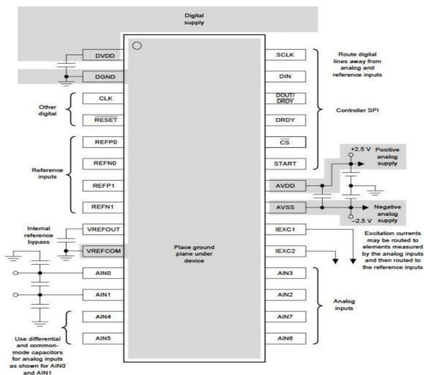
图46. ADSD1247布局案例
