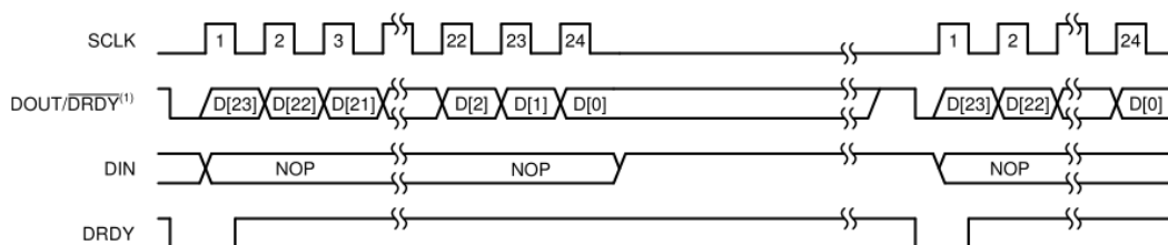
图21.DRDY 模式位=1时的数据检索(使能)
