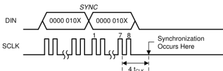
图25.同步命令操作
