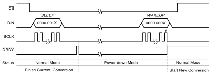
图24.睡眠和唤醒命令操作
