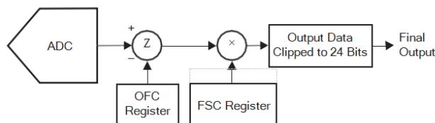
图19.校准框图
