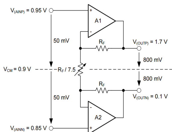
图9 VCM 处于最低限值的示例
