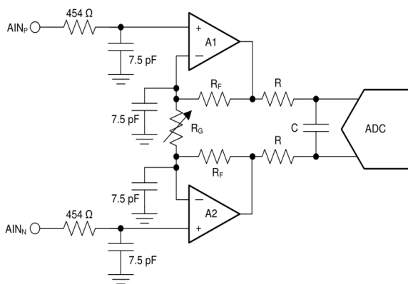
图7.PGA的简图
