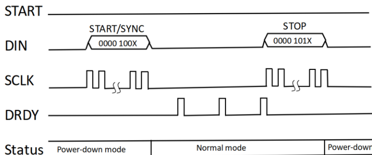
图 18.退出启动/同步命令控制模式
