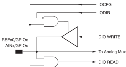
图 13.模拟和数据接口引脚
