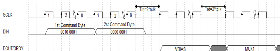
图30a.从寄存器读取 (SCLK频率1Mhz及以上时序)
