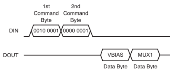
图30b.从寄存器读取 (SCLK频率1Mhz及以下时序)
