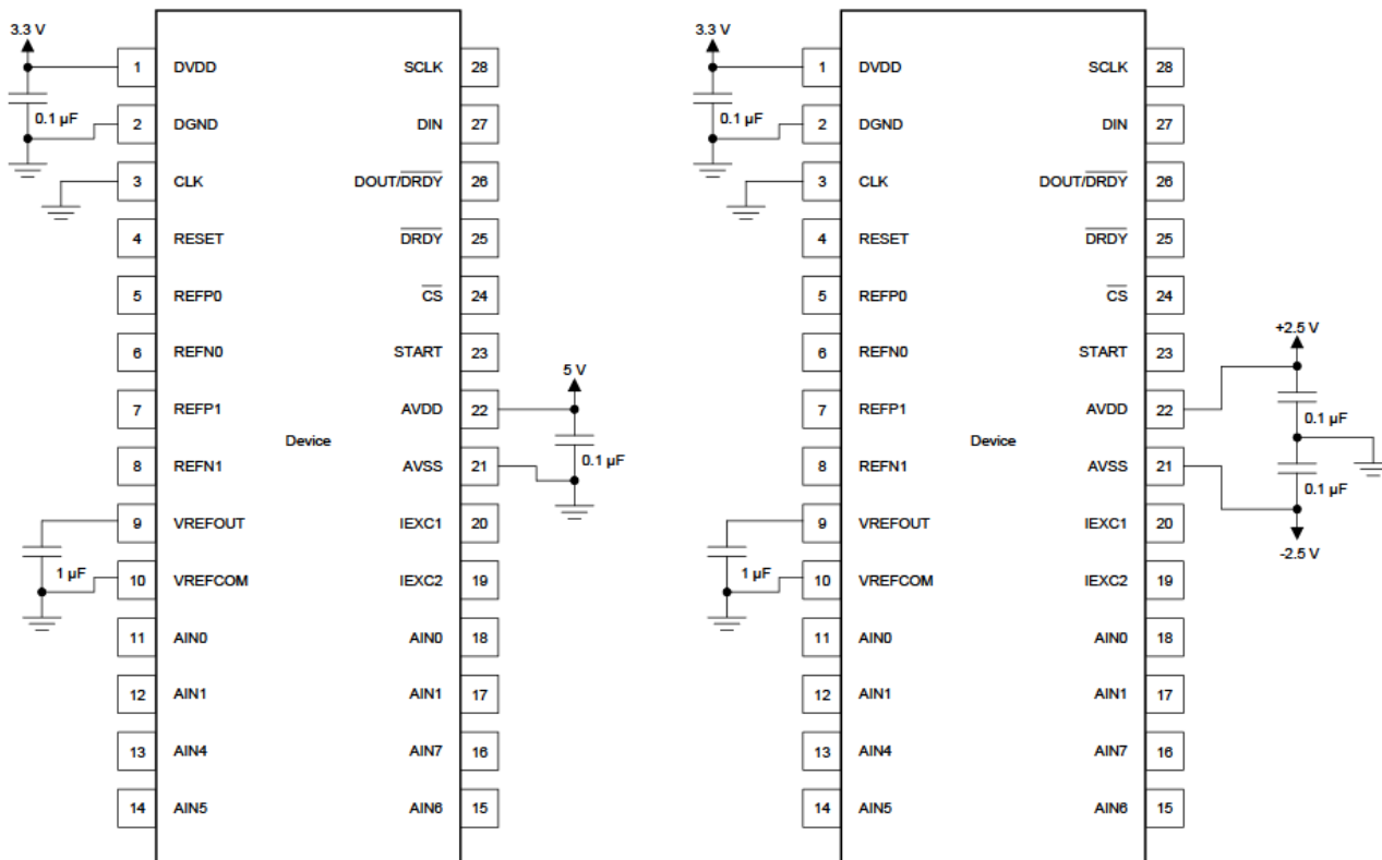
图45. 单极和双极电源运行的电源去耦
