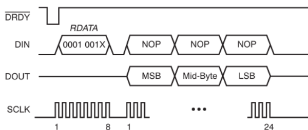
图 27.读取数据一次
