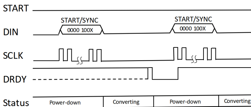
图 16.使用 START/SYNC 命令的单次转换时序
